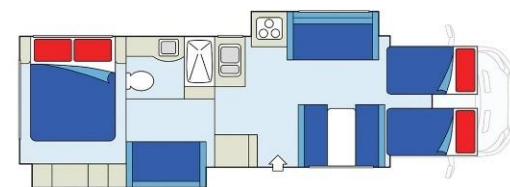
Maxi-plus Motorhome MH-X
