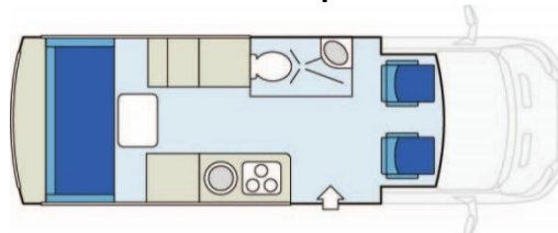
Deluxe Van Camper DVC
